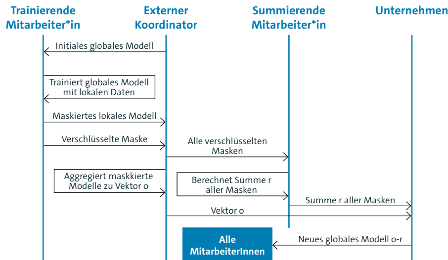
Abbildung 7: Privatsphäre währendes föderiertes Lernen. Mitarbeiter*innen stellen zuerst fest (nicht im Bild), ob sie trainierende oder summierende Mitarbeiter*innen sind, oder ob sie keinen Beitrag dazu leisten. Trainierende Mitarbeiter*innen berechnen aus dem globalen Modell und lokalen Daten ein neues lokales Modell und schicken ihr maskiertes lokales Modell sowie die Verschlüsselung der Maske an den Koordinator. Der Koordinator schickt die Verschlüsselungen der Masken an summierende Mitarbeiter*innen, die sie entschlüsseln, die Summe aller Masken berechnen und diese an das Unternehmen schicken. Der Koordinator schickt die Aggregation aller maskierten lokalen Modells an das Unternehmen. Das Unternehmen berechnet aus diesen erhaltenen Vektoren das globale Modell und schickt es allen Mitarbeiter*innen zur weiteren Verwendung.
