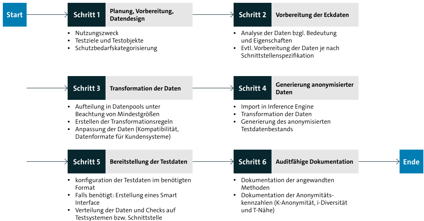
Abbildung 15: Ablauf bei Semantischer Anonymisierung für Testdaten
