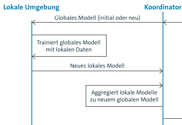
Abbildung 6: Schematische Darstellung einer Runde des föderierten Lernens. Zuerst sendet der Koordinator an lokale Umgebungen ein neues globales KI-Modell. Anschließend trainieren die lokalen Umgebungen mit lokalen Daten dieses erhaltene globale Modell. Die daraus resultierenden neuen lokalen Modelle werden jeweils an den Koordinator geschickt. Der Koordinator aggregiert die erhaltenen lokalen Modelle zu einem neuen globalen Modell und schickt es an lokale Umgebungen, um eine weitere Runde des föderierten Lernens einzuleiten.
