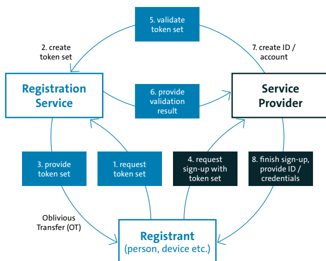
Abbildung 1: Funktionsweise des PAUTH-Verfahrens
