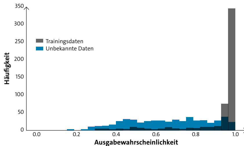
Abbildung 11: Verteilungen der Ausgabewahrscheinlichkeiten nach Trainings- und unbekannten Referenzdaten (jeweils 500 Datenpunkte) auf Purchase 10 Datensatz. Eigene Erstellung.
