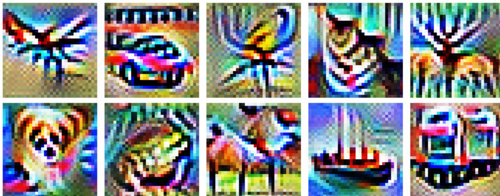
Abbildung 8: Model Inversion Angriff auf den CIFAR 10 Datensatz, in Anlehnung an [2]. Die rekonstruierten Klassen sind: Oben – Flugzeug, Auto, Vogel, Katze, Hirsch. Unten – Hund, Frosch, Pferd, Schiff, LKW.
