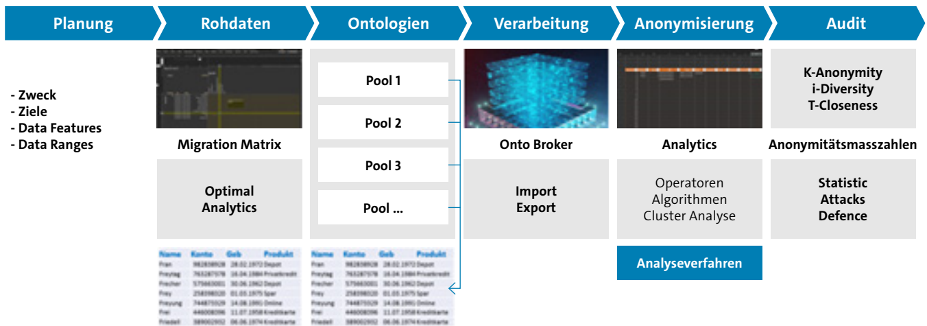
Abbildung 13: Abfolge der Schritte bei Semantischer Anonymisierung
