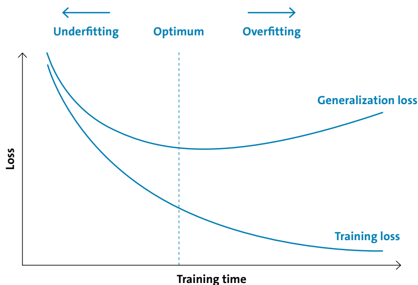
Abbildung 10: Zusammenhang Training loss und Generalisierungsfähigkeit, in Anlehnung an: Zhang, Lipton, Li, Smola, Dive into Deep Learning, 2019 [7].
