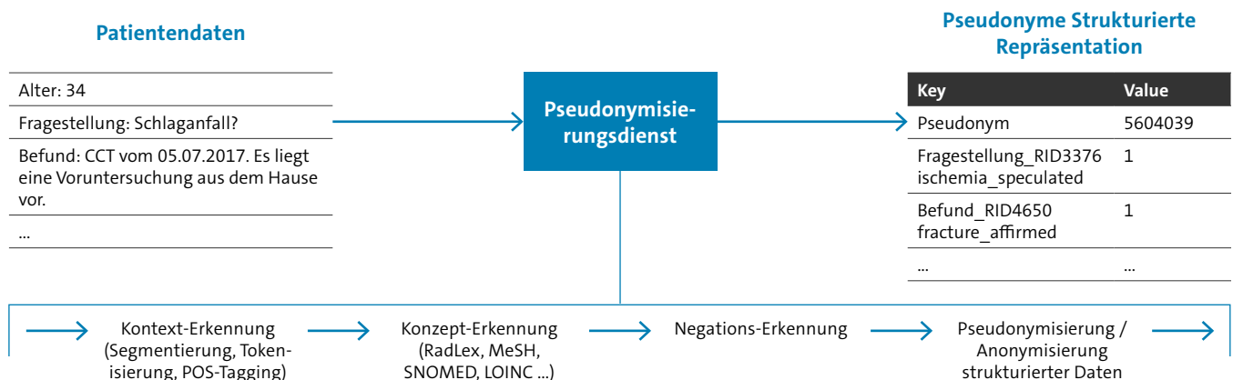
Abbildung 12: Umsetzungsvorschlag »Pseudonymisierungsdienst«
